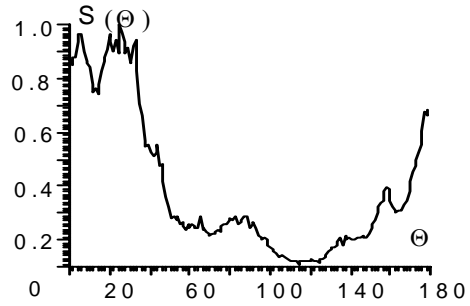
Рис. 1. Определение преимущественного направления водных потоков: а - фрагмент космического снимка участка устья реки Днепр, б график азимутального распределения ПЧС изображения.
